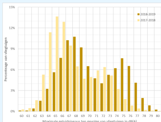
figuur 46: maximale geluidsniveaus tijdens een vliegtuigpassage boven Villawijk
