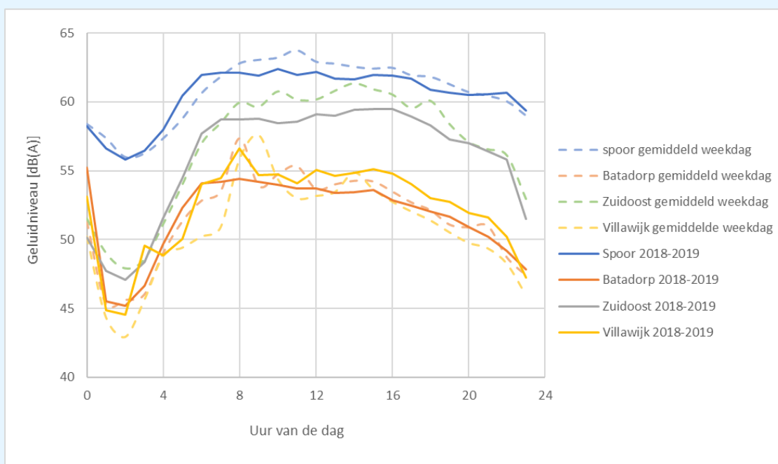
figuur 10: weekdaggemiddelde voor 2018-2019 (doorgetrokken lijn) en gemiddelde over afgelopen 7 jaar (stippellijn) Zie boven
