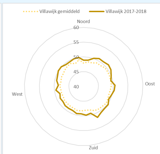
figuur 60: geluidsniveaus als functie van windrichting voor locatie Zuidoost
