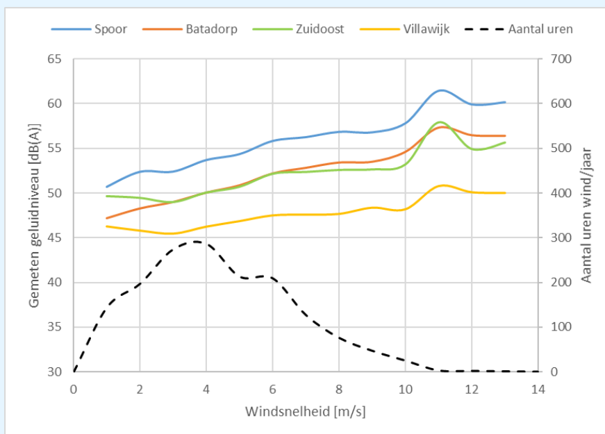
figuur 55: overzicht gemeten geluidsniveau (verticale as links) als functie van windsnelheid (horizontale as) bij zuidwestenwind op de verschillende meetlocaties. Eveneens weergegeven is het aantal uren gedurende de meetperiode dat een bepaalde windsnelheid voorkwam (verticale as rechts). De waarden zijn gemiddeld op basis van uurgemiddelde windsnelheden en uurgemiddelde geluidsniveaus.
