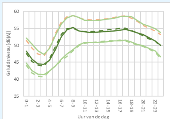
figuur 31: variatie in geluidsniveau locatie: Zuidoost, de bovenste lijn is de 90 percentiel, middelste lijn de 50 percentiel en de onderste lijn de 10 percentiel (de doorgetrokken lijn = 2018-2019, gestippelde lijn - gemiddelde 2012-2019)
