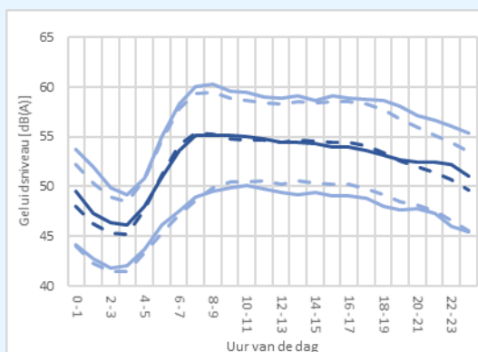
figuur 29: variatie in geluidsniveau locatie: Spoor, de bovenste lijn is de 90 percentiel, middelste lijn de 50 percentiel en de onderste lijn de 10 percentiel (de doorgetrokken lijn = 2018-2019, gestippelde lijn - gemiddelde 2012-2019)
