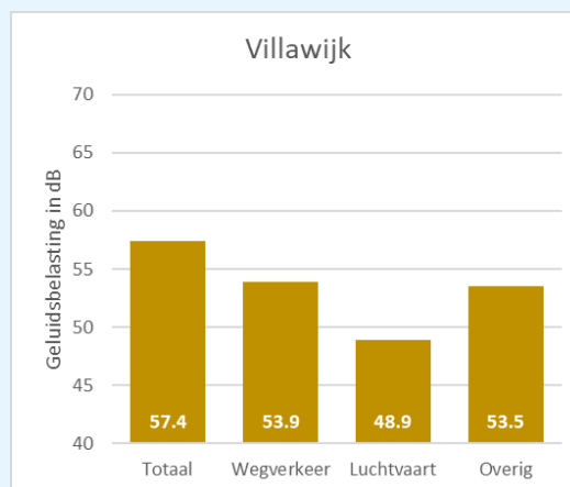
Figuur 64: opsplitsing totaalgeluid naar bronsoort locatie Villawijk
