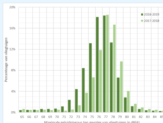
figuur 47: maximale geluidsniveaus tijdens een vliegtuigpassage boven Zuidooost
