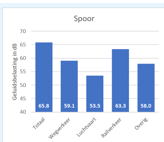
figuur 12: opsplitsing totaalgeluid naar bronsoort locatie Spoor
