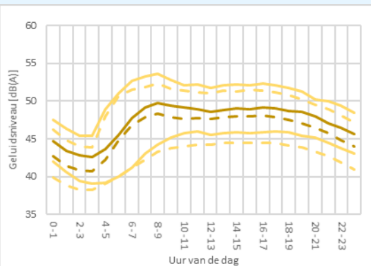
figuur 32: variatie in geluidsniveau locatie: Villawijk, de bovenste lijn is de 90 percentiel, middelste lijn de 50 percentiel en de onderste lijn de 10 percentiel (de doorgetrokken lijn = 2018-2019, gestippelde lijn - gemiddelde 2012-2019)
