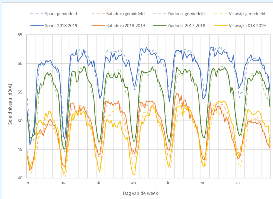
figuur 11: verloop van geluid over dagen van de week. Gemiddelde voor 2018-2019 (doorgetrokken lijn) en gemiddelde over afgelopen zes jaar (stippellijn) per locatie.
