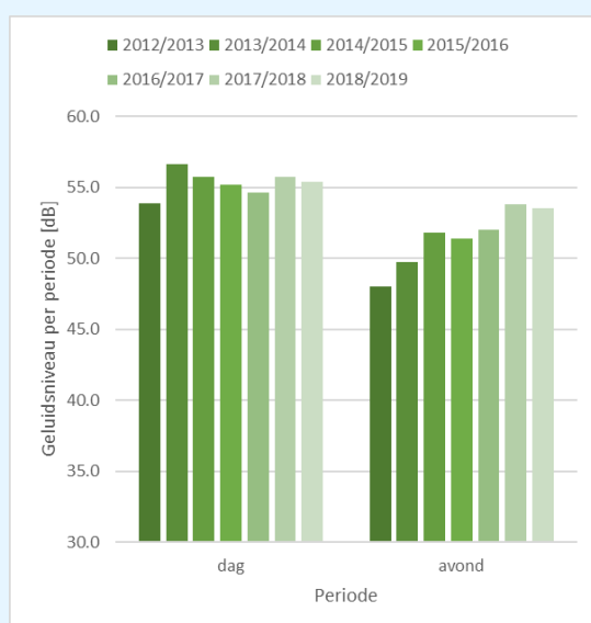
figuur 44: verloop geluidsniveau luchtvaart overdag en 's avonds locatie Zuidoost
