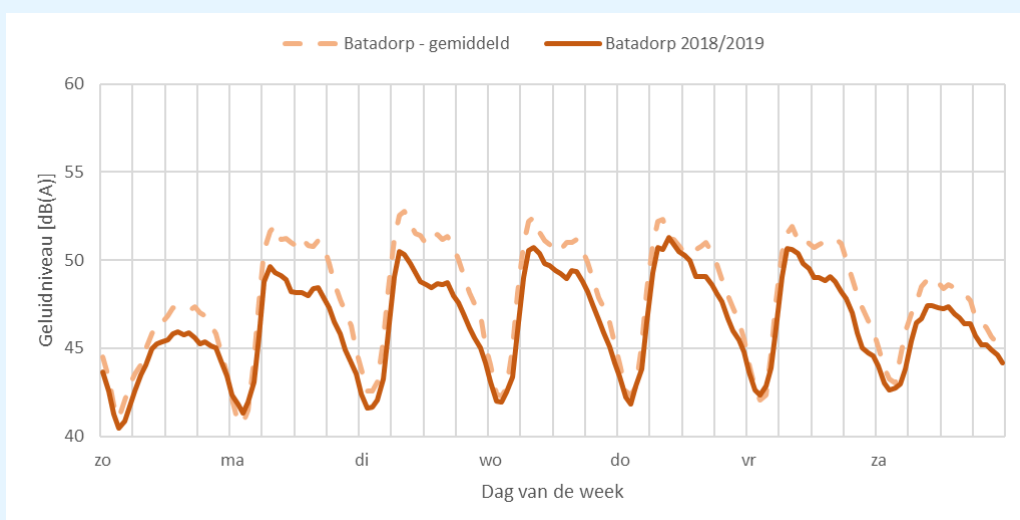
figuur 25: gemiddeld geluidsniveaupercentage van wegverkeer gedurende de week voor locatie Batadorp (lineair gemiddeld)
