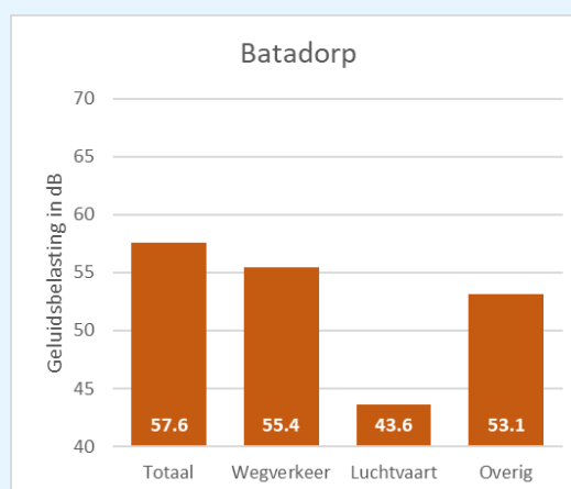
Figuur 62: opsplitsing totaalgeluid naar bronsoort locatie Batadorp
