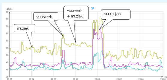
figuur 52: Housequake (op 12 mei 2012) met westenwind (beige Zuidoost, paars Villawijk, Blauwgroen Batadorp)
