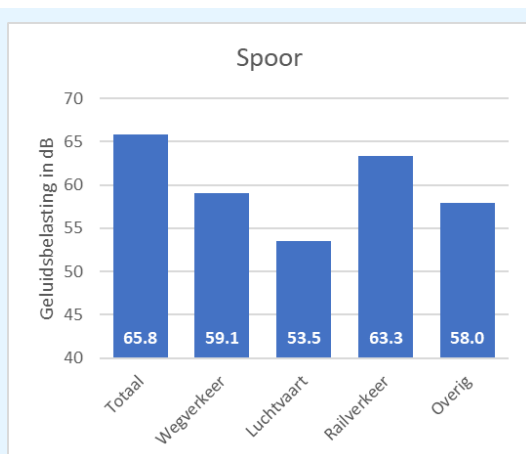
figuur 61: opsplitsing totaalgeluid naar bronsoort locatie Spoor
