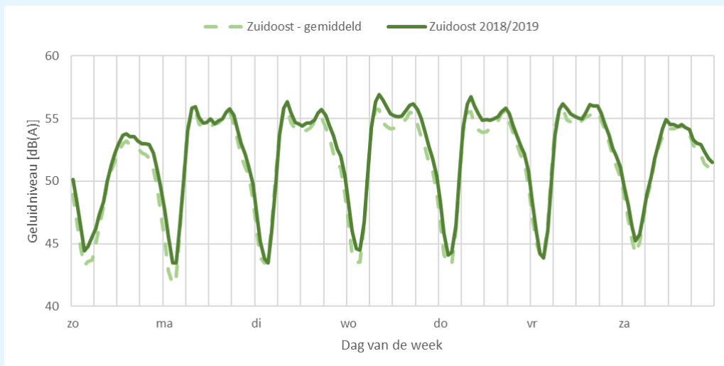
figuur 26: gemiddeld geluidsniveauverloop van wegverkeer gedurende de week voor locatie Zuidoost. Hierin is te zien het geluidsniveau gedurende meetperiode 2018-2019 (doorgetrokken lijn) en het gemiddelde van de meetperiodes ervoor (stippellijn) (lineair gemiddeld)
