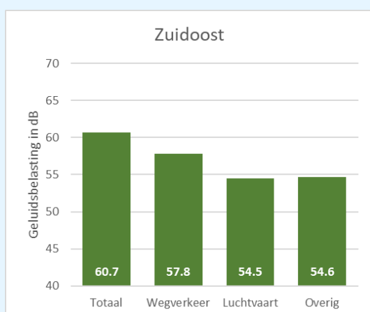
figuur 14: opsplitsing totaalgeluid naar bronsoort locatie Zuidoost
