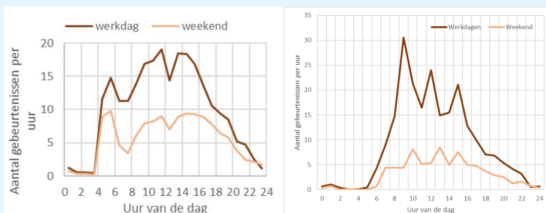
figuur 51: links: Batadorp aantal piekniveaus boven de 60 dB(A) (uit rapportage 2015-2016). Rechts: Batadorp aantal piekniveaus boven de 60 dB(A) in meetjaar 2018/2019
