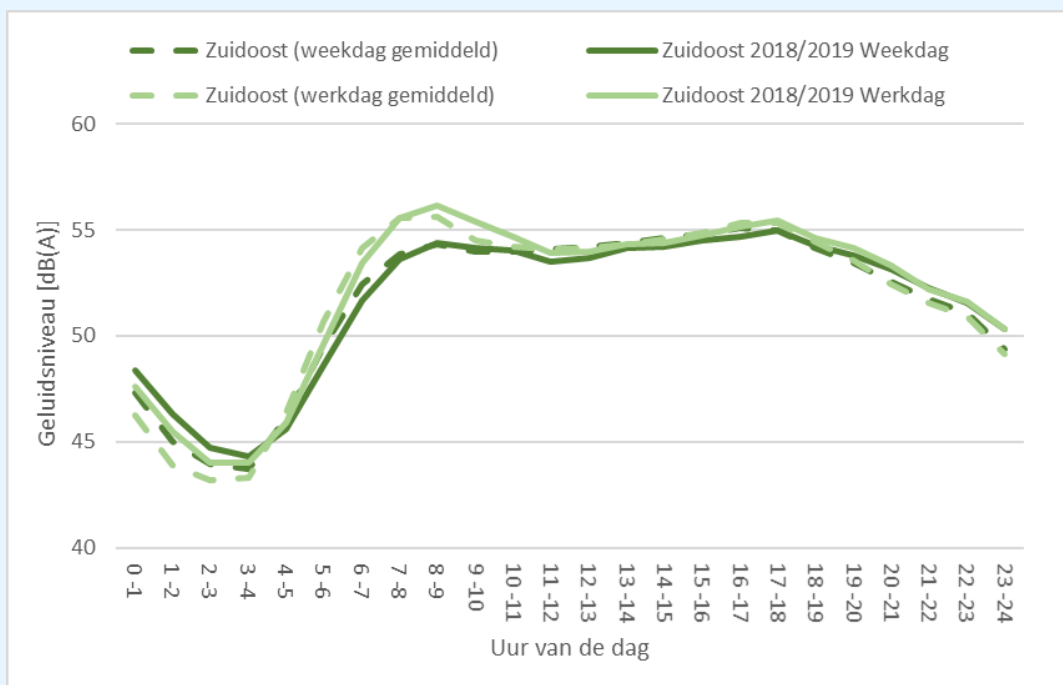
figuur 22: werkdag gemiddelden (lichte kleur) en weekdag gemiddelden (donkere kleur) voor de laatste meetperiode en gemiddeld over afgelopen 7 jaar voor de locatie Zuidooost (lineair gemiddeld)
