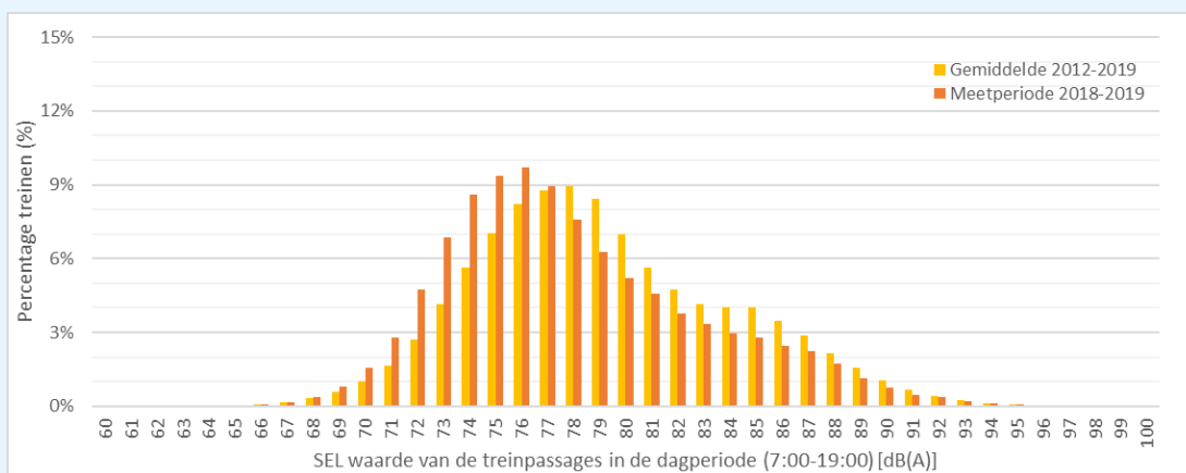
figuur 37: spreiding in maximale geluidsniveaus van treinpassages in de dagperiode
