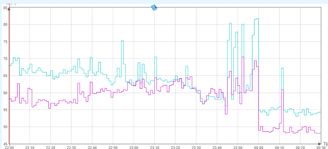
figuur 54: Lakedance (op 11 augustus 2018) met noordwesten wind en vuurwerk net voor twaalfen (turquoise Zuidoost en paars Villawijk)
