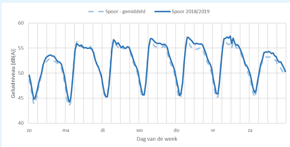
figuur 24: gemiddeld geluidsniveaupercentage van wegverkeer gedurende de week voor locatie Spoor. Hierin is te zien het geluidsniveau gedurende meetperiode 2018-2019 (doorgetrokken lijn) en het gemiddelde van de meetperiodes ervoor (stippellijn) (lineair gemiddeld)
