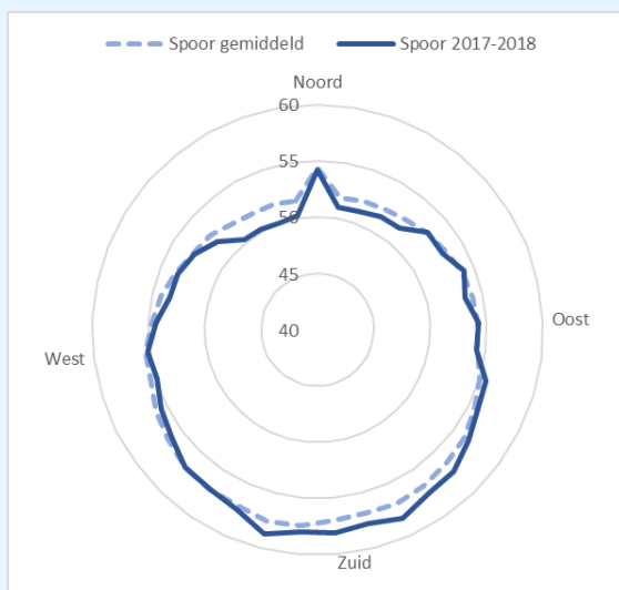
figuur 57: geluidsniveaus als functie van windrichting voor locatie Spoor
