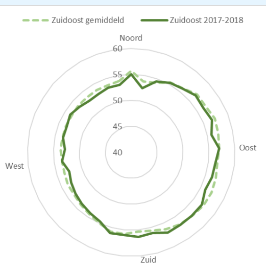
figuur 58: geluidsniveaus als functie van windrichting voor locatie Zuidoost
