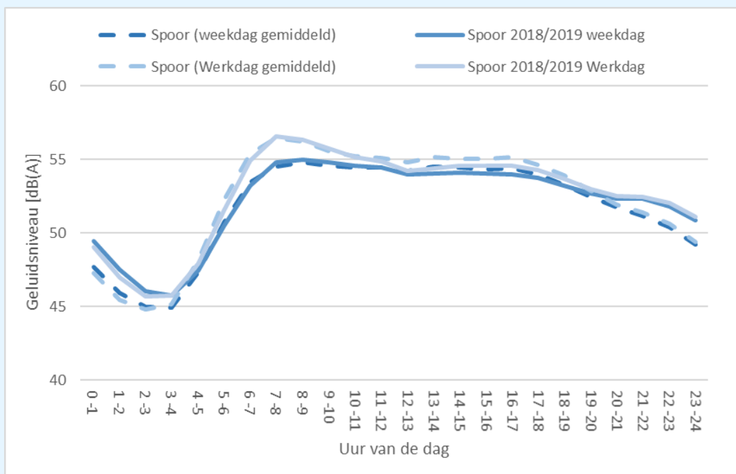
figuur 20: werkdag gemiddelden (lichte kleur) en weekdag gemiddelden (donkere kleur) voor de laatste meetperiode en gemiddeld over afgelopen 7 jaar voor de locatie Spoor (lineair gemiddeld)
