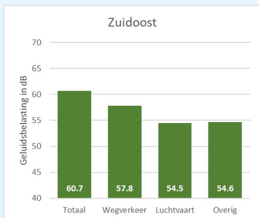
Figuur 63: opsplitsing totaalgeluid naar bronsoort locatie Zuidoost
