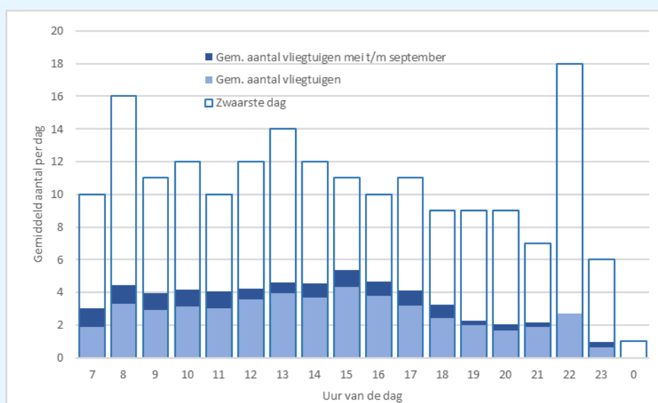
figuur 49: aantal vliegtuigen per uur op de meetlocatie Villawijk
