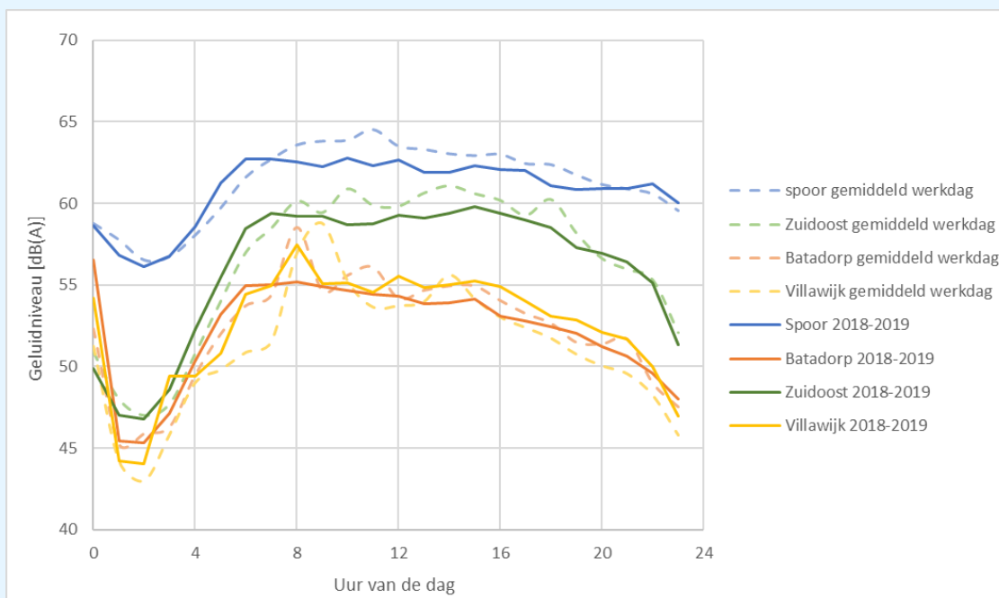
figuur 9: werkdaggemiddelde voor 2018-2019 (doorgetrokken lijn) en gemiddelde over afgelopen 7 jaar (doorgetrokken lijn)
