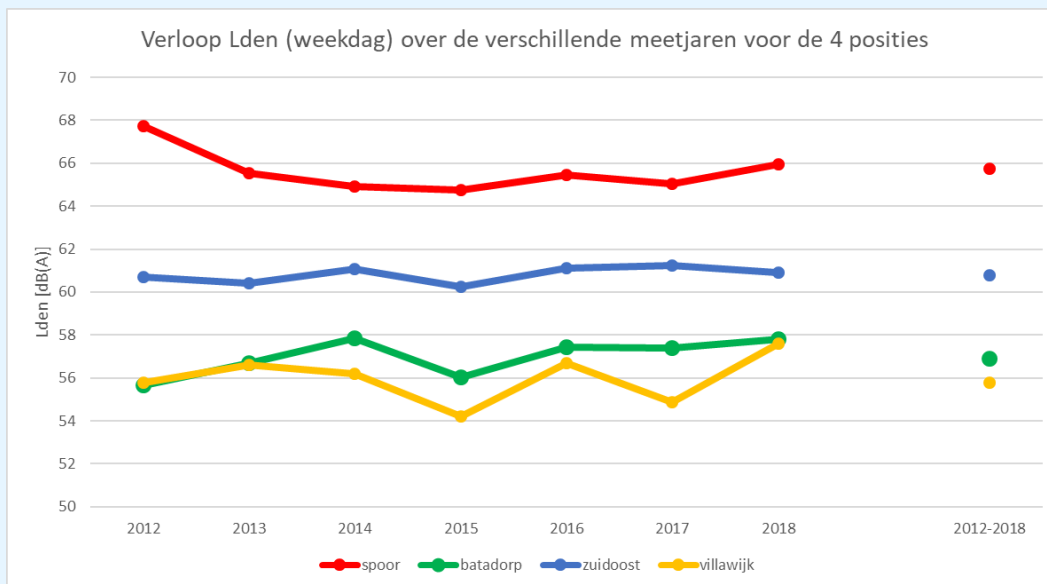
figuur 8: verloop van het gemeten L den op de 4 meetlocaties voor de afgelopen 7 jaar (rechts het gemiddelde over 7 jaar meten)
