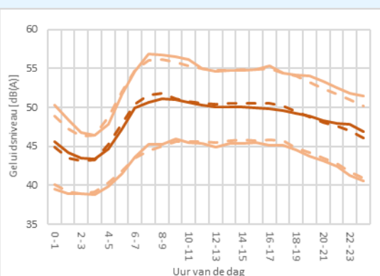
figuur 30: variatie in geluidsniveau locatie: Batadorp, de bovenste lijn is de 90 percentiel, middelste lijn de 50 percentiel en de onderste lijn de 10 percentiel (de doorgetrokken lijn = 2018-2019, gestippelde lijn - gemiddelde 2012-2019)
