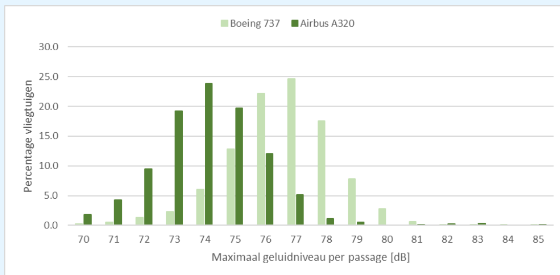
figuur 48: verschil in maximale geluidsniveaus voor de Boeing 737 en Airbus A320
