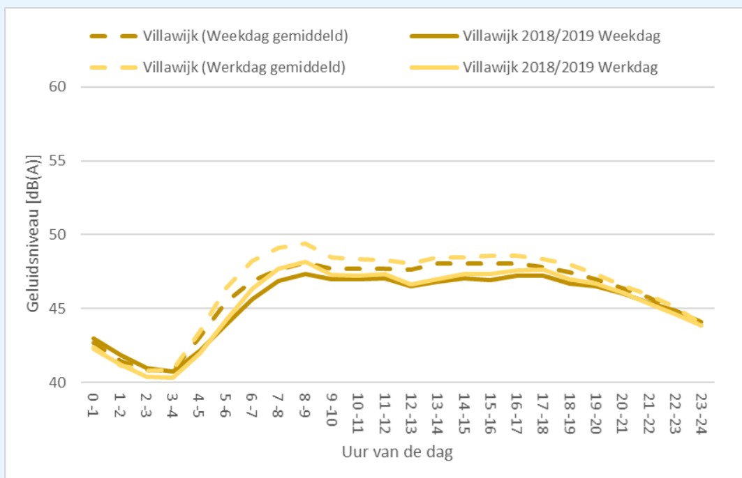
figuur 23: werkdag gemiddelden (lichte kleur) en weekdag gemiddelden (donkere kleur) voor de laatste meetperiode en gemiddeld over afgelopen 7 jaar voor de locatie Villawijk (lineair gemiddeld)
