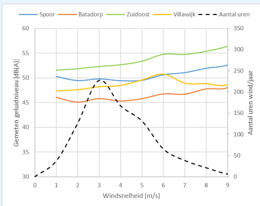
figuur 56: overzicht gemeten geluidsniveau (verticale as links) als functie van windsnelheid (horizontale as) bij noordoostenwind op de verschillende meetlocaties. Eveneens weergegeven is het aantal uren gedurende de meetperiode dat een bepaalde windsnelheid voorkwam (verticale as rechts). De waarden zijn gemiddeld op basis van uurgemiddelde windsnelheden en uurgemiddelde geluidsniveaus
