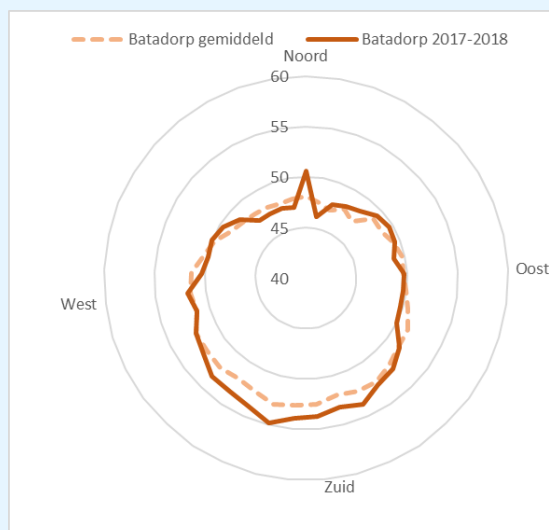
figuur 59: geluidsniveaus als functie van windrichting voor locatie Batadorp
