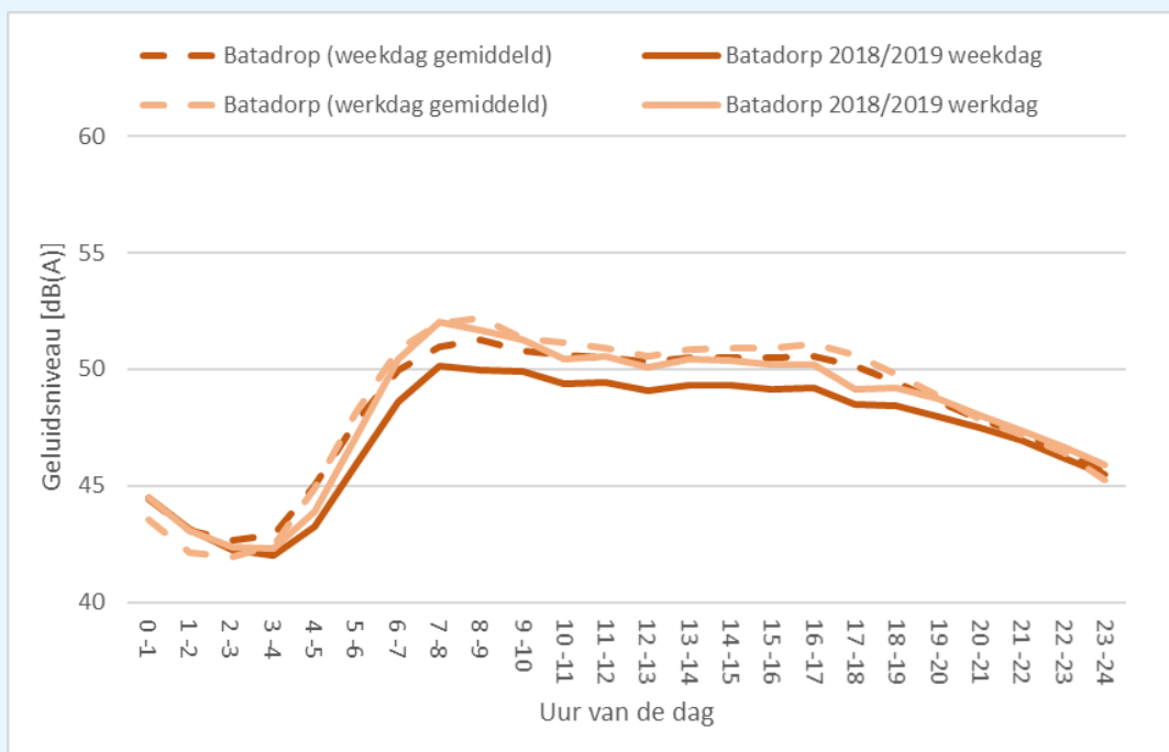
figuur 21: werkdag gemiddelden (lichte kleur) en weekdag gemiddelden (donkere kleur) voor de laatste meetperiode en gemiddeld over afgelopen 7 jaar voor de locatie Batadorp (lineair gemiddeld)
