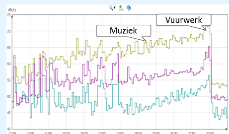
figuur 53: Lakedance (op 11 augustus 2012) met oostenwind (beige Zuidoost, paars Villawijk, Blauwgroen Batadorp)
