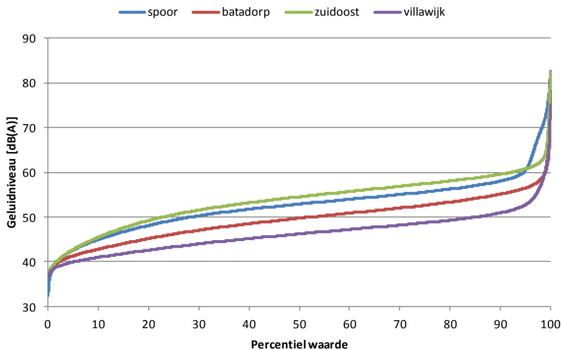
Figuur 33: Percentiel waarden in 2014
