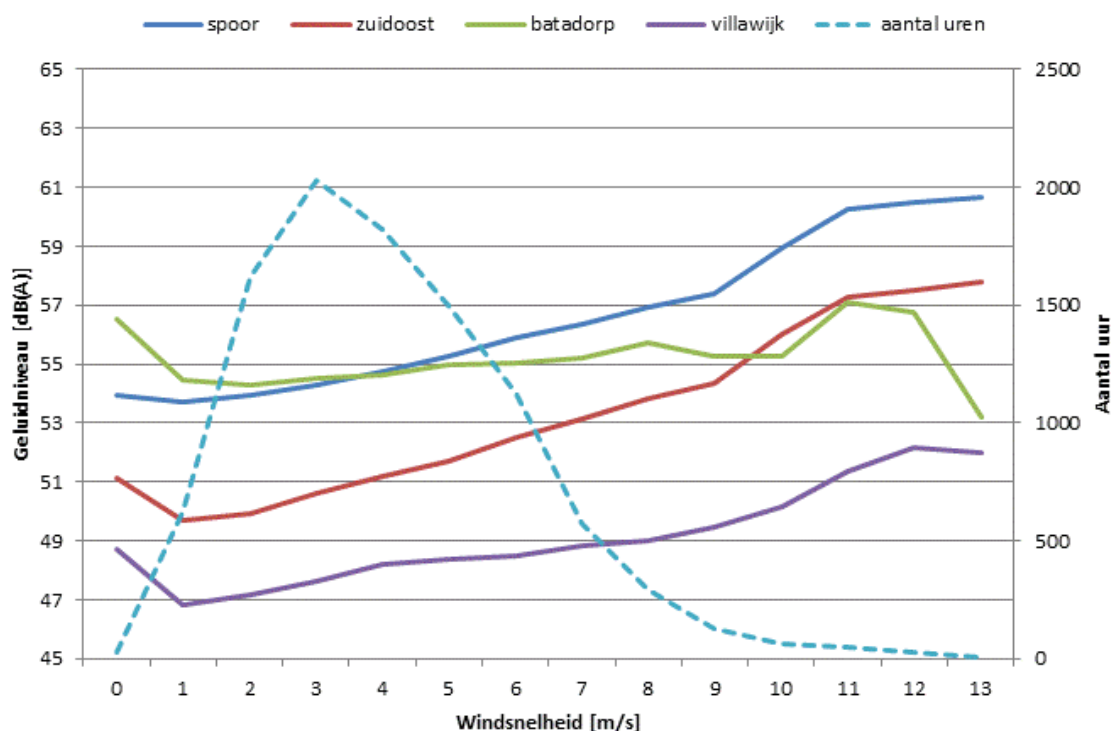
Figuur 30: overzicht gemeten als functie van windsnelheid. Tevens weergegeven is het aantal uren gedurende de meetperiode dat een bepaalde windsnelheid voorkwam. De waarden zijn gemiddeld op basis van uurgemiddelde windsnelheden en uurgemiddelde geluidsniveaus.
