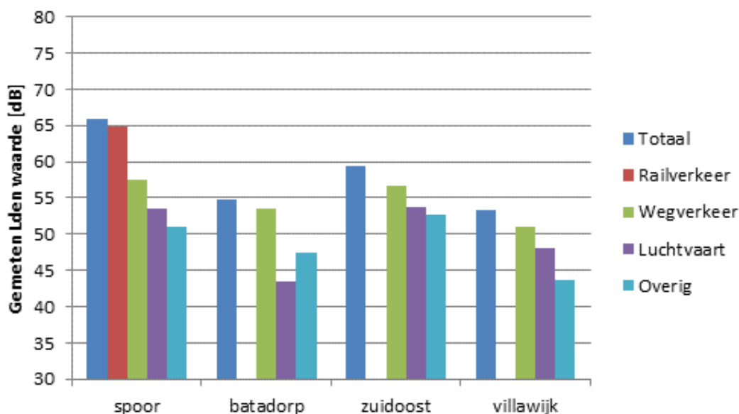
Figuur 39: overzicht totale L_{den} -waarden en de deelbijdragen per bron. Overige bronnen zijn niet herkend.
