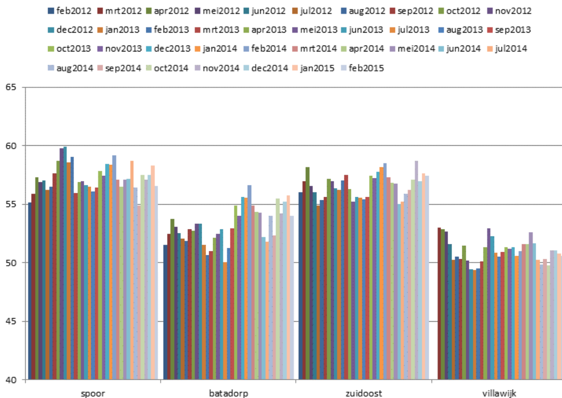
Figuur 10: gemeten L_{den} -waarden wegverkeer per maand. Ter hoogte van meetpunt villawijk zijn geen meetgegevens beschikbaar over de maand februari 2012.
