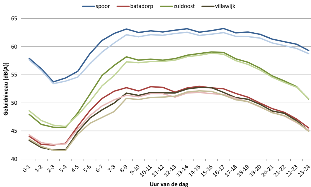
Figuur 6: weekgemiddeld uurverloop gedurende een dag
