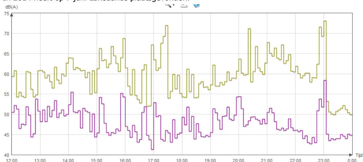
Figuur 28: overzicht gemeten geluidsniveaus van Lakedance voor locatie zuidoost (beige) en villawijk (paars)
