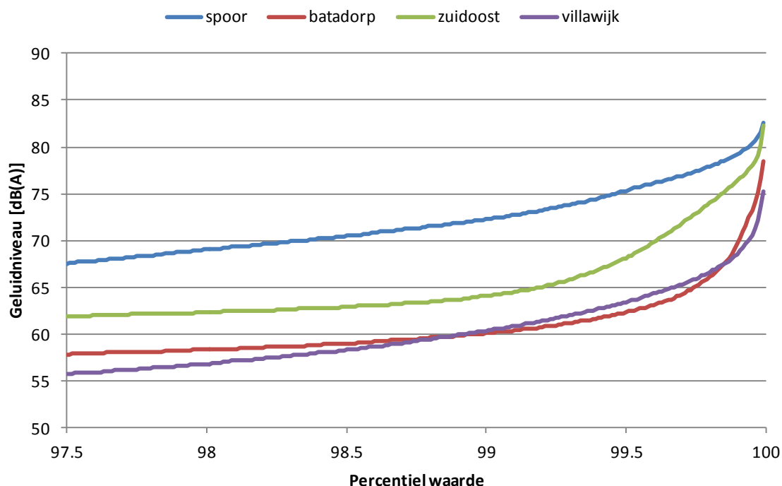
Figuur 34: Percentiel waarden in 2014
