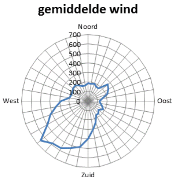
Figuur 32: overzicht aantal uren gedurende de dagperiode en over de meetperiode dat een bepaalde windrichting voorkwam. Er is gekeken in stappen van 10 graden (36 windrichtingen).
