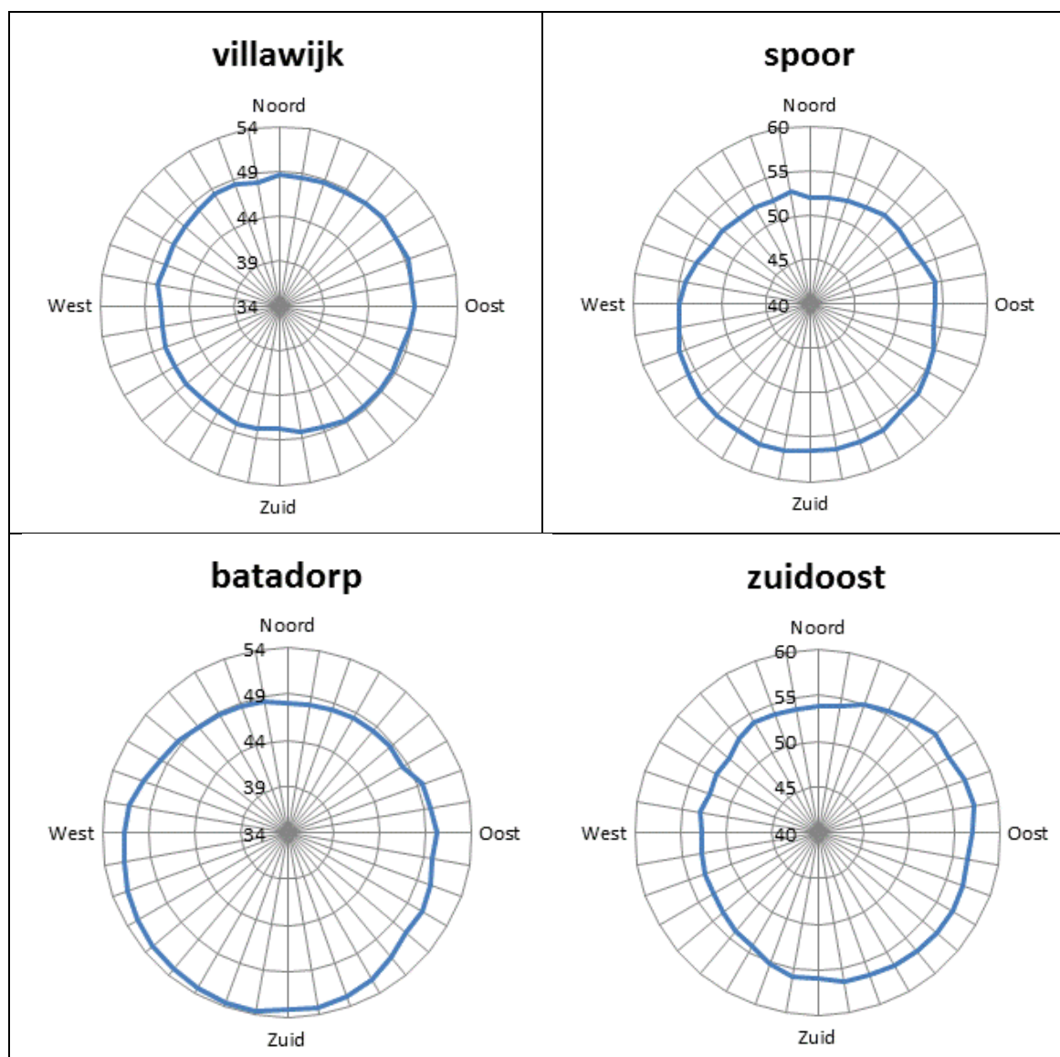
Figuur 31: overzicht gemiddeld geluidsniveau van wegverkeer tussen 07.00 en 19.00 als functie van windrichting. Metingen zonder of bij veranderlijke wind is buiten beschouwing gelaten.
