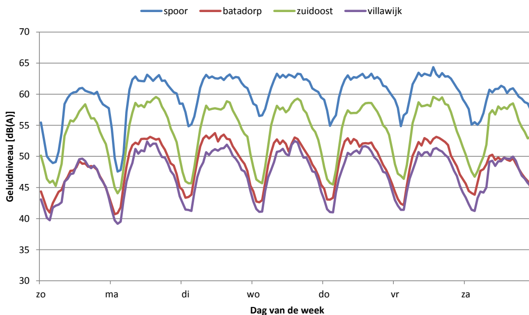
Figuur 7: overzicht gemiddelde geluidsniveaus gedurende een week
