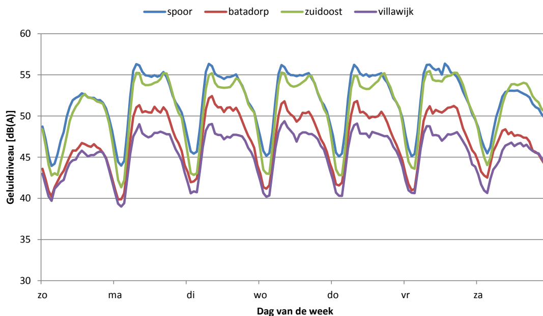
Figuur 9: overzicht geluidsniveaus wegverkeer gedurende een week
