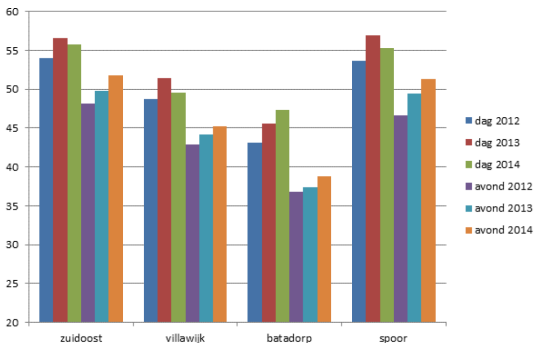
Figuur 17: verschil geluidniveaus in de dag en avondperiode voor 2012, 2013 en 2014
