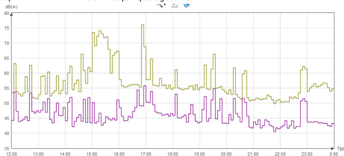
Figuur 29: overzicht gemeten geluidsniveaus van Winterpark voor locatie zuidoost (beige) en villawijk (paars)
