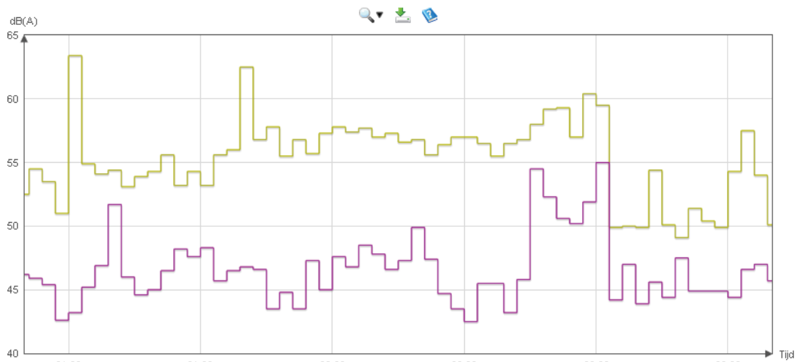
Figuur 22: overzicht gemeten geluidsniveaus rond het einde van Lakedance voor locatie Zuidooost (beige) en villawijk (paars)
