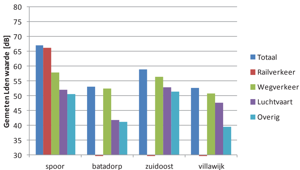
Figuur 5: overzicht totale L_{den} waarden en de deelbijdragen per bron. Overige bronnen zijn niet herkend (zie uitleg in komende hoofdstukken).
