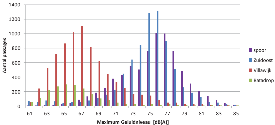
Figuur 18: overzicht spreiding in maximale geluidsniveaus tussen vliegtuigpassages
