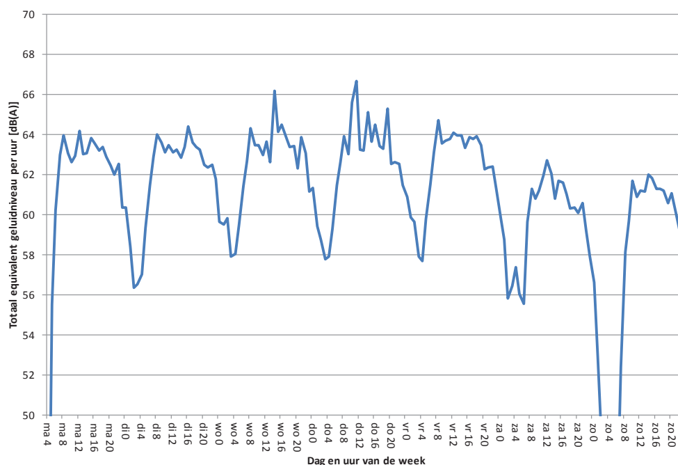
Figuur 13: verloop equivalent geluidsniveau per uur gedurende een week
