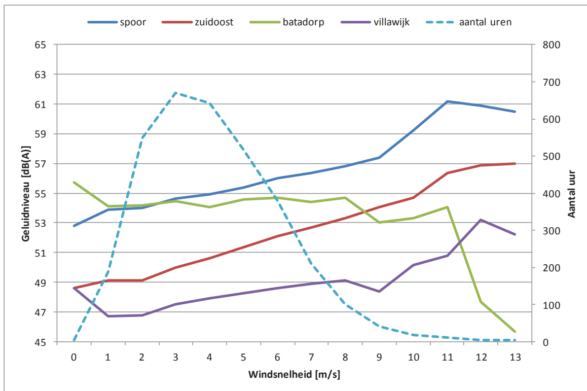
Figuur 26: overzicht gemeten als functie van windsnelheid. Tevens weergegeven is het aantal uren gedurende de meetperiode dat een bepaalde windsnelheid voorkwam. De waarden zijn gemiddeld op basis van uurgemiddelde windsnelheden en uurgemiddelde geluidsniveaus.
